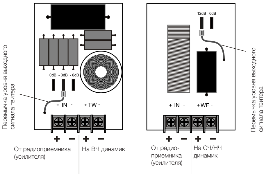
Рисунок 6 Схема подключения кроссовера
